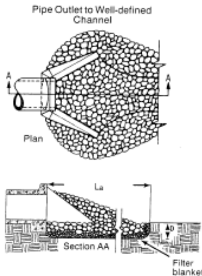
Figure 7-4 Riprap Apron
